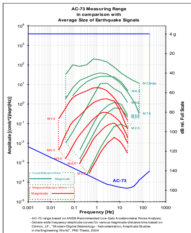
Диапазон измерения AC-73-DH по сравнению с типичными уровнями сигналов локальных и региональных землетрясений
